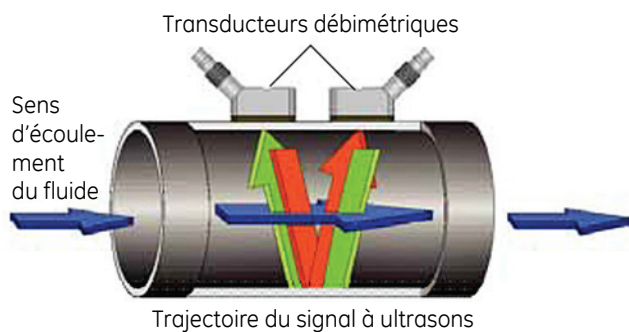
Technique de mesure du débit à temps de transit
